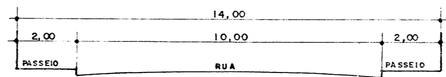
PERFIL TRANSVERSAL DAS RUAS
